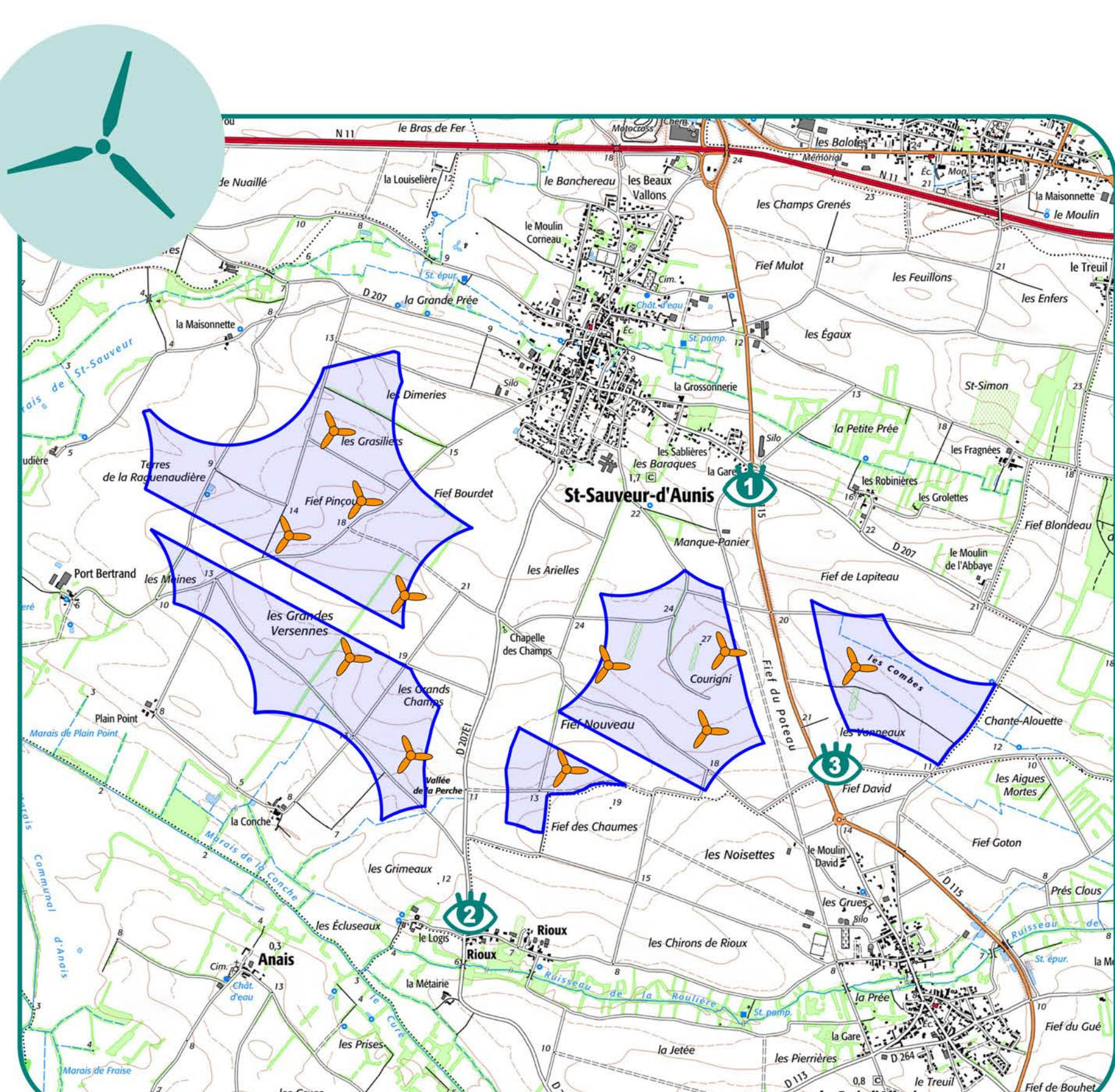
Variante n°1 11 éoliennes
