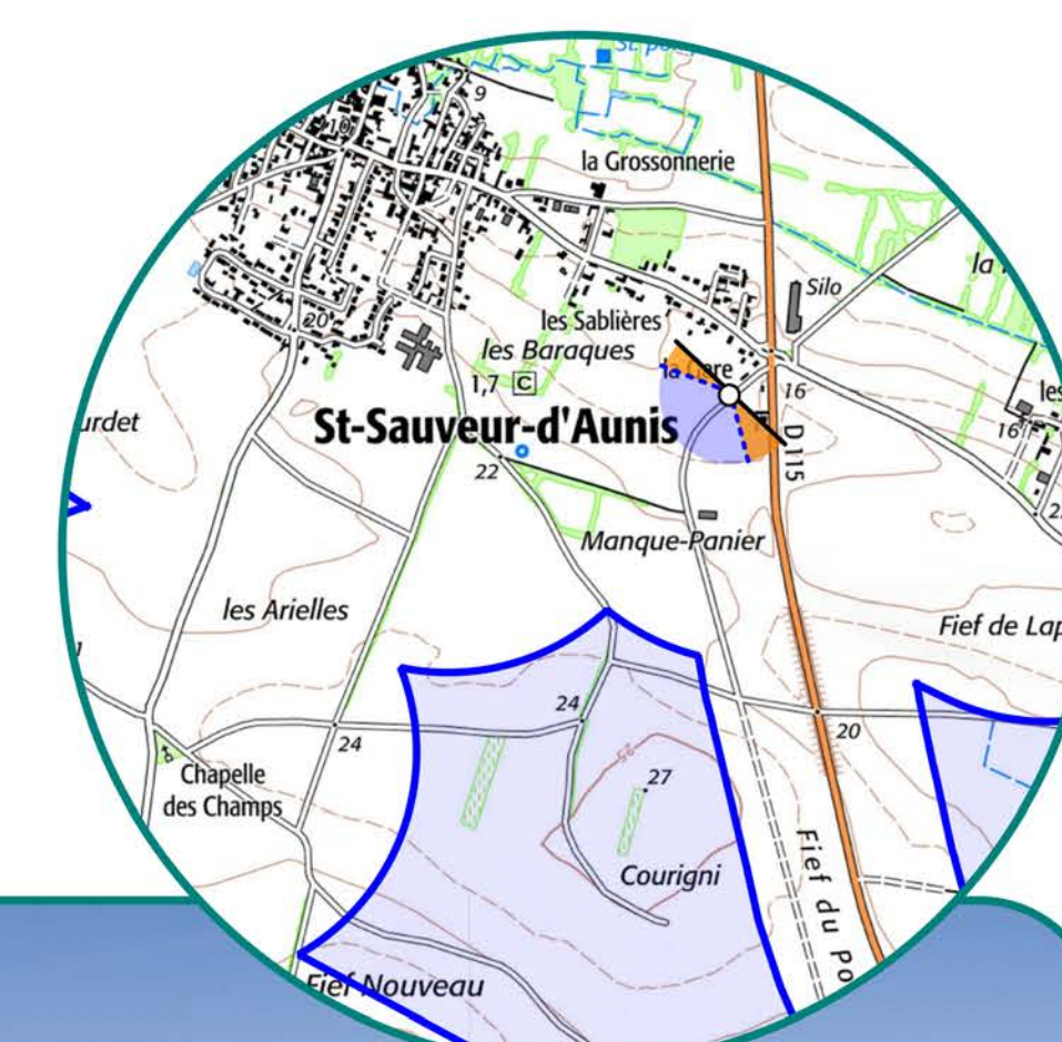
Variante n°3 (retenu) 8 éoliennes
